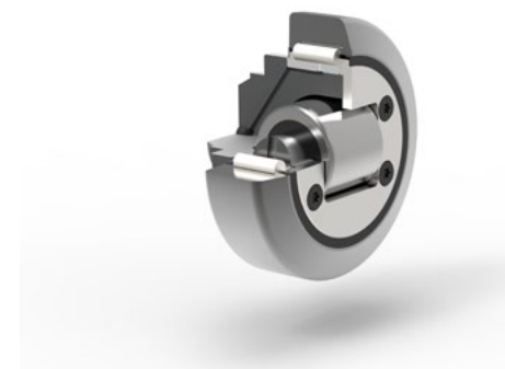
Axialrolle fest ➡ 132-137
