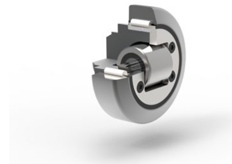
Axialrolle justierbar über Exzenter ➡ 120-125
