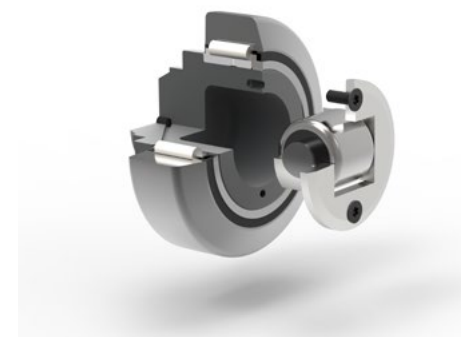
Axialrolle justierbar über Distanzierscheiben ➡ 126-131
