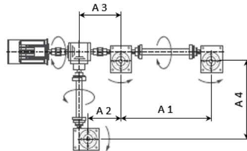
Anordnung 8
