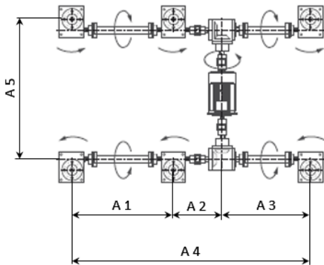
Anordnung 5
