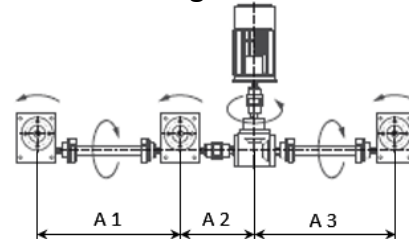
Anordnung 10
