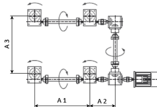
Anordnung 10
