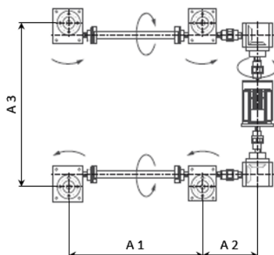
Anordnung 9
