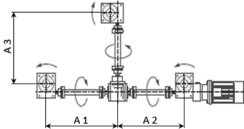
Anordnung 5
