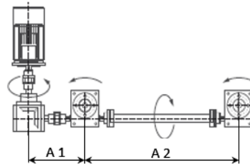
Anordnung 4
