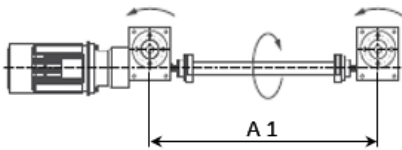
Anordnung 1
