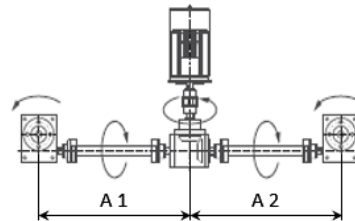
Anordnung 6
